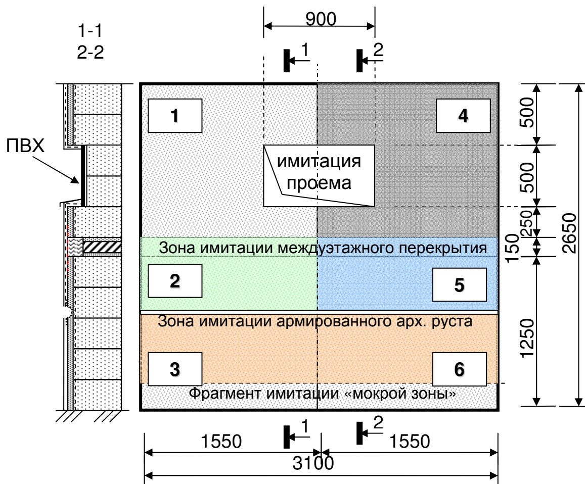
Рис. 3. Схема фрагмента стены из газобетонных блоков с защитно-декоративной отделкой Ceresit
