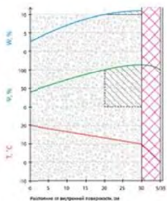
B1 – мокрое утепление по ППС 50/100 мм
