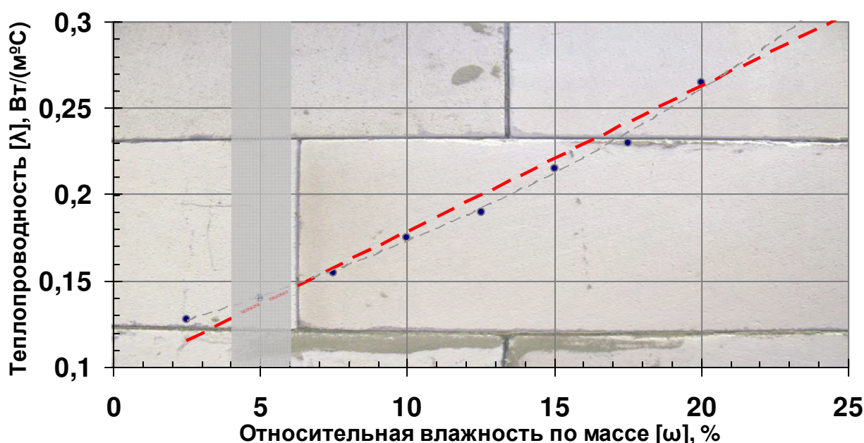
Рис. 1. График линейной зависимости теплопроводности от влажности для автоклавного газобетона марки D 500
