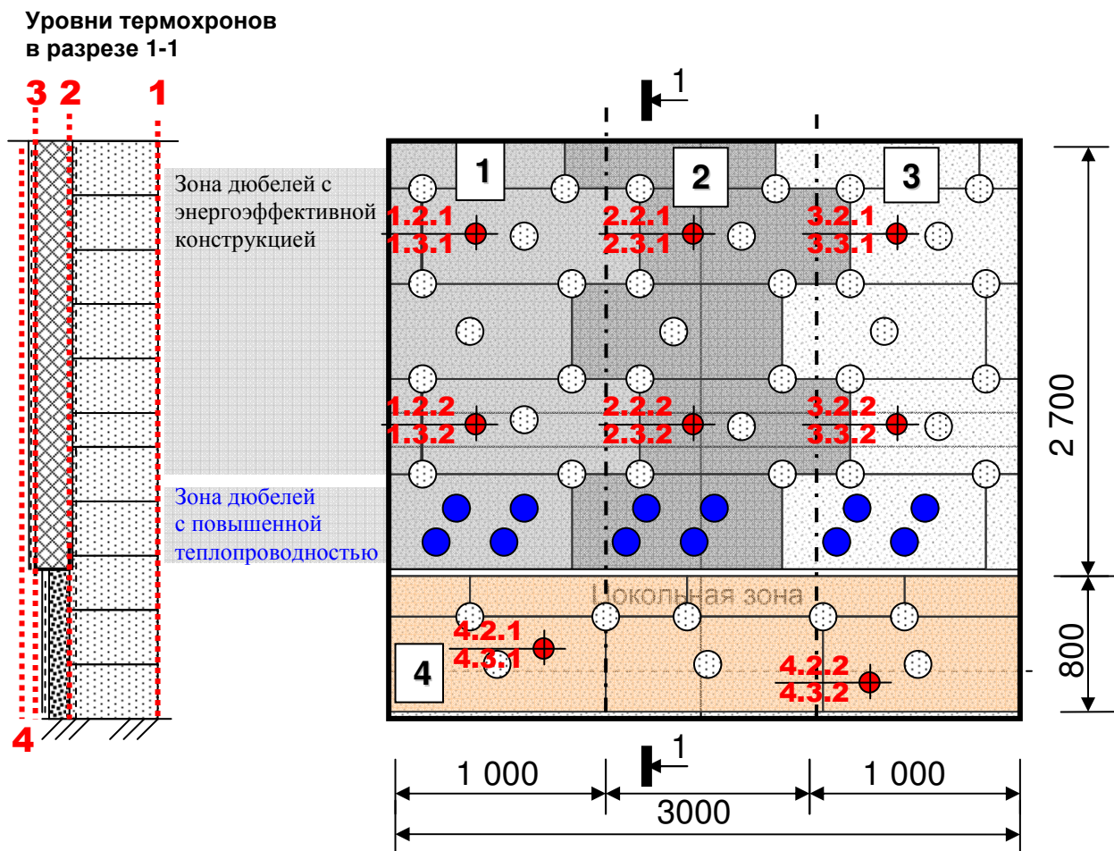
Рис. 4. Схема фрагмента стены из газобетонных блоков с наружной теплоизоляцией и защитно-декоративной отделкой Ceresit
