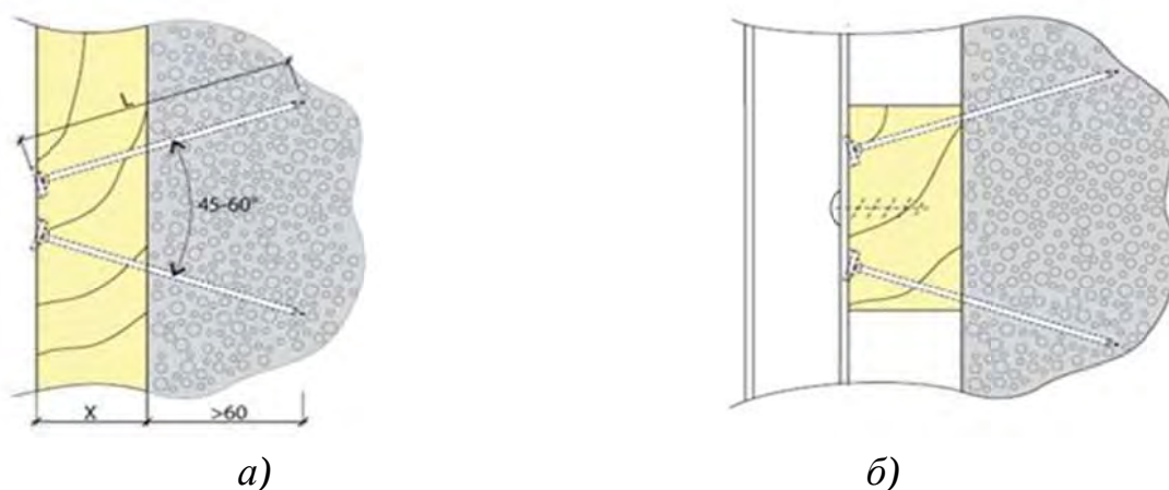
Рис. 12. Гвоздевое крепление обрешетки: а — деревянный брус, набитый на кладку непосредственно; б — крепление профиля через опорный брусок
