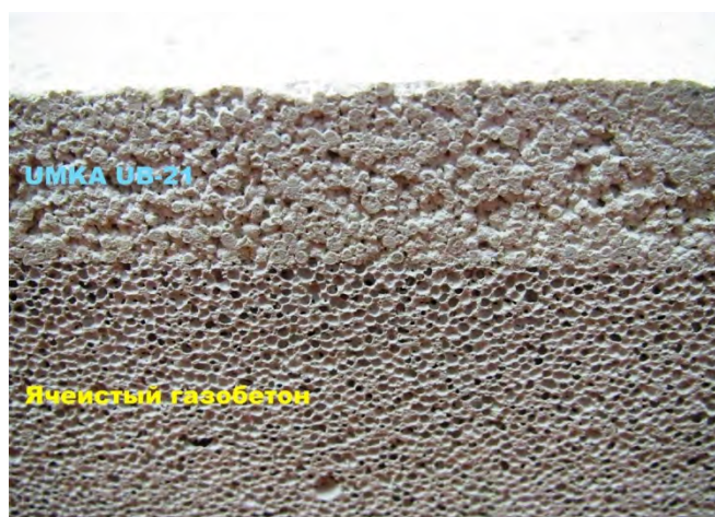
Рис. 1. Макросъемка среза штукатурного слоя УМКА UB-21, нанесенного на газобетон.
