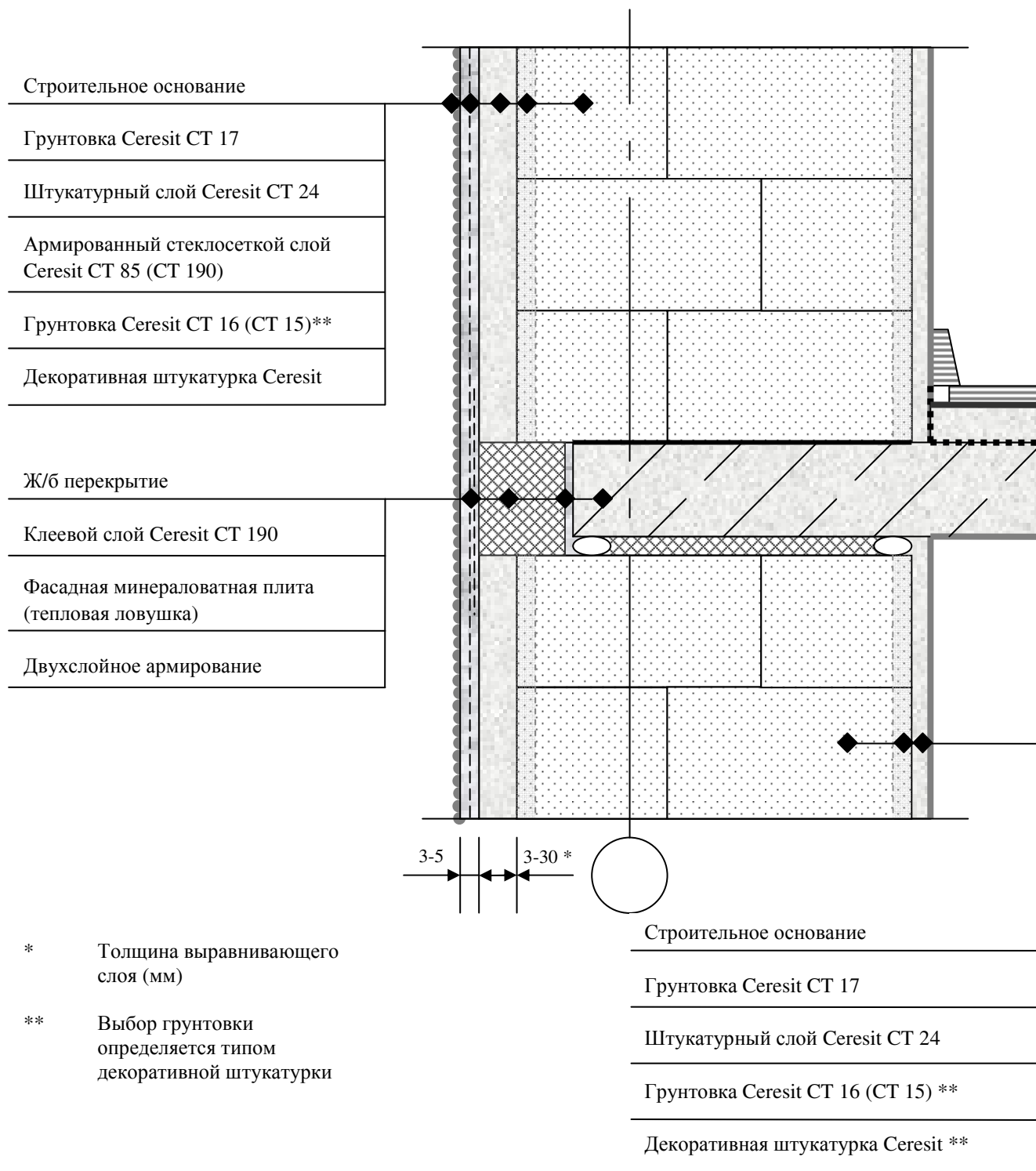
Рис. 2. Фрагмент стены из газобетонных блоков с защитно-декоративной отделкой Ceresit
