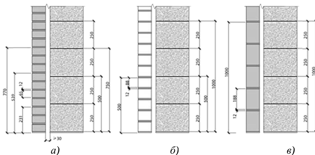
Рис. 15. Двухслойные кладки с облицовками:
