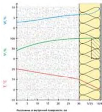
B1 – мокрое утепление по минвате 50/
