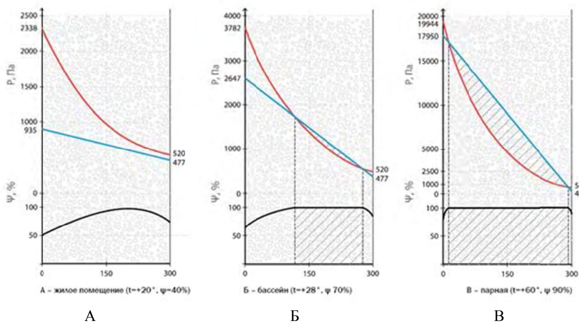
Рис. 26. Влияние микроклимата на распределение влажности воздуха в порах по толщине стены: А – жилое помещение (t = 20°, Ψ = 40%); Б – бассейн (t = 28°, Ψ = 70%); В – баня (t = 60°, Ψ = 90%).
